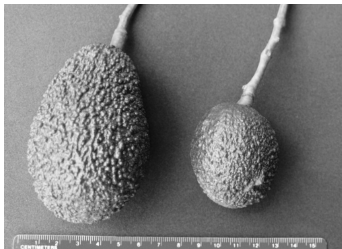
FIGURA 1. Frutos de aguacate 'Hass' seis meses después del amarre, tomados de árboles tratados con ZnSO_4 al suelo (izquierda), comparado con el fruto pequeño y redondo (derecha) de los árboles sin ZnSO_4 .
