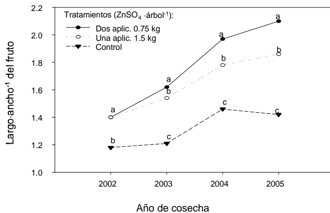
FIGURA 3. Efecto anual de las aplicaciones de ZnSO_4 al suelo sobre la forma del fruto (relación largo/ancho) en aguacate 'Hass'. Medias con la misma letra para cada año son iguales estadísticamente (Duncan, P \leq 0.05 ).
