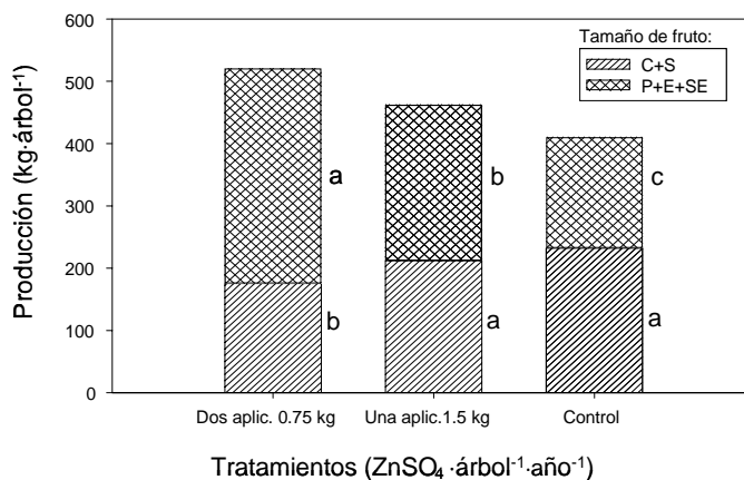
FIGURA 2. Efecto de la aplicación de ZnSO_4 al suelo en árboles de aguacate 'Hass' sobre la producción acumulada de fruto (cosechas 2003, 2004 y 2005) y su distribución según el tamaño del fruto: grandes (Primera + Extra + Súper extra; P + E + SE) y pequeños (Canica + Segunda; C+S). Medias con la misma letra para cada grupo de tamaño de fruto son iguales estadísticamente (Duncan, P \leq 0.05 ).
