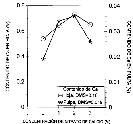
Figura 1. Efecto de la concentración de nitrato de calcio asperjado foliarmente (seis aplicaciones) sobre el contenido de calcio en hojas y pulpa de aguacate ( Persea americana Mill.) cv. Hass. Diferencia mínima significativa (DMS) de acuerdo a la prueba de Tukey al 5% de probabilidad.
